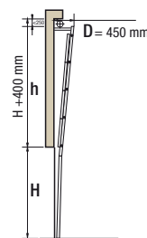
VL – Vertikala takskenor
