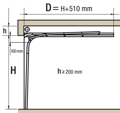
LHR-FM – torsionsfjäder monterad fram.
