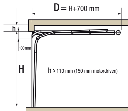
LHR-RM – torsionsfjäder monterad bak.
